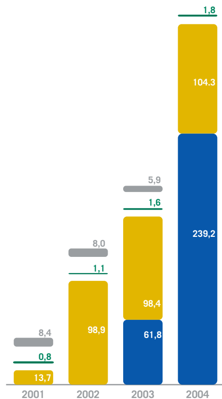
Tratamiento aguas servidas Gran Santiago (millones de m 3 )
